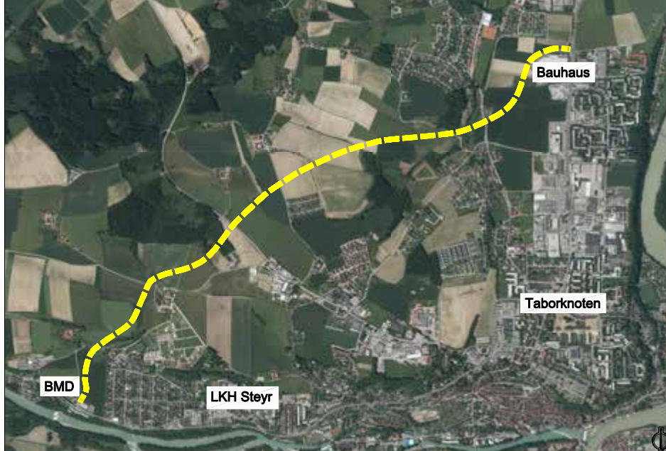
Die Trassierung der Steyrer Westspange, die bis 2021 verwirklicht werden soll.
