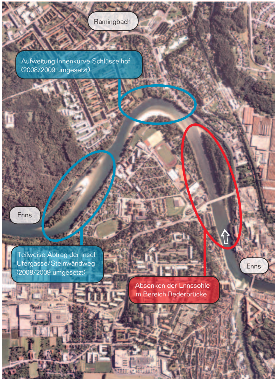
Das Bild zeigt die bereits verwirklichten Hochwasserschutz-Maßnahmen (blau markiert) und die vorgesehene 3. Ausbaustufe des Hochwasserschutz-Projektes, die Enns-Fluss-Eintiefung (rot markiert).
